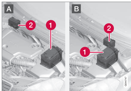
А: Лівостороннє кермо. В: Правостороннє кермо. (1) Акумулятор стартера 16 (2) Допоміжний акумулятор.
