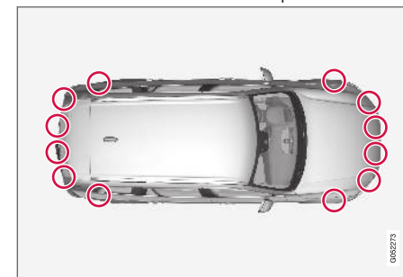
Parkeringssensoreernas placering 119 .
