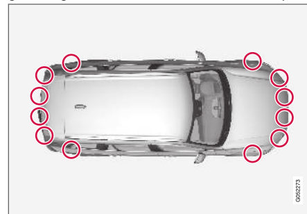
Parkeringssensorernas placering 133 .
