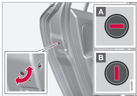
Manuell låsning av dörr. Ej att förväxlas med Barnsäkerhetsspärr (s. 175).
