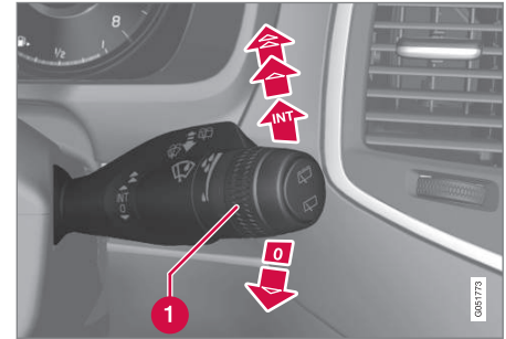
Rechter stuurhendel.
