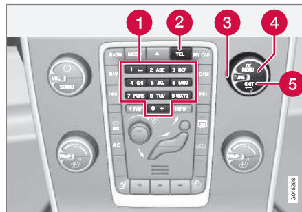
Panneau de commande dans la console centrale.
