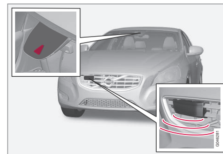
Caméra et capteur radar 1
