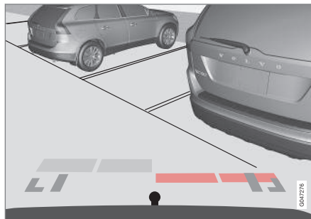
Les marqueurs teintés (à raison d'un marqueur par capteur) indiquent la distance.
