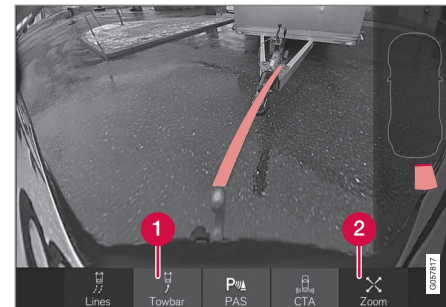
Crochet d'attelage avec ligne indicatrice.
