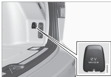
Gniazdo elektryczne 12 V w przestrzeni bagażowej*.
