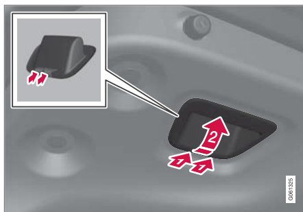
行李廂蓋關閉把手。
