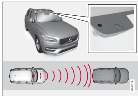
攝影機與雷達單元測量與前車的距離 47 。
