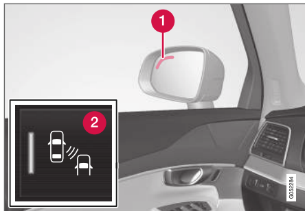
Positie van het BLIS-lampje 72 .
