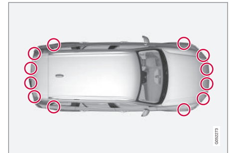
PAP-tunnistimien sijainti 27 .
