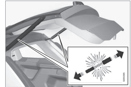
Sähkötoimisen takaluukun esiäjännitetyt jouset.
