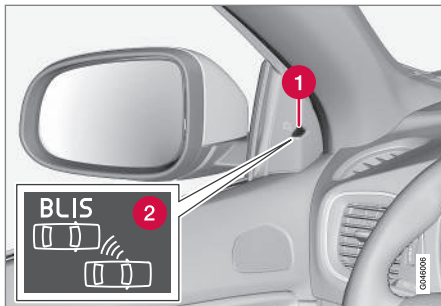
Positie BLIS-lampje 36 .
