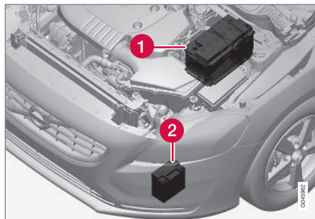
(1) Startaccu 15 (2) Hulpaccu
