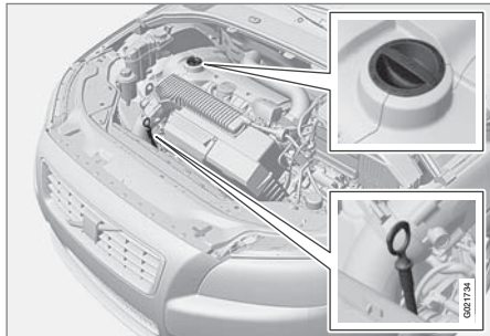
オイルレベルゲージおよびフィラーパイプ
