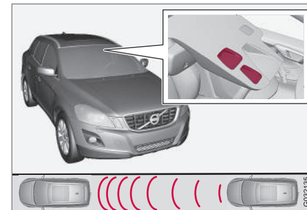
Emplacement du capteur laser dans le pare-brise 6
