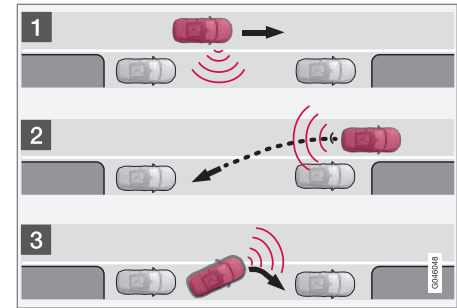
Principio de PAP.
