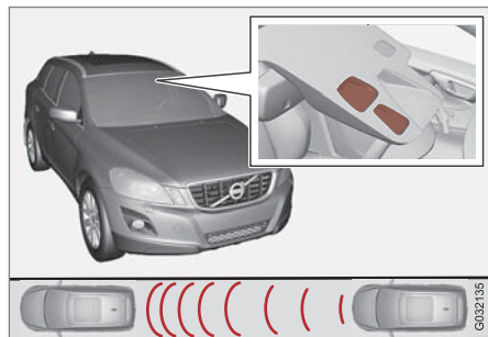
レーザーセンサーの送信/受信ウィンドウ 18
