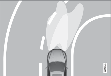
アクティブヘッドライトを解除したときの照射パターン(左)と作動したときの照射パターン(右)
