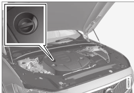
Påfyllingsrør 13 .
