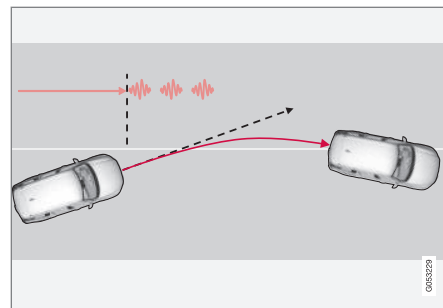
A Assistência de faixa de rodagem avisa através de vibração no volante 7 .
