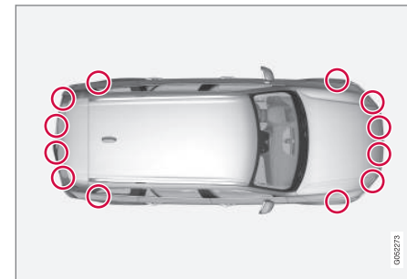
Localização dos sensores PAP.
