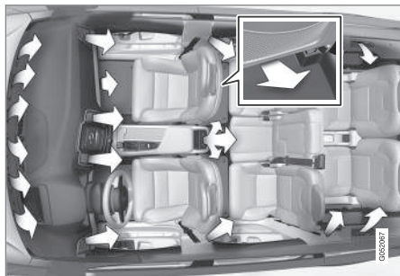
Distribuição de ar no habitáculo com climatização de 4 zonas.
