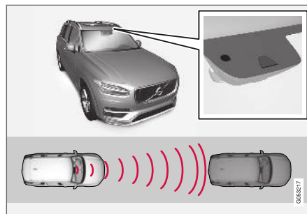
Umiejscowienie modułu radarowego 81 .
