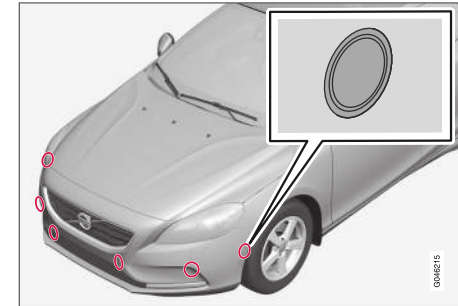
Датчики PАР расположены в бамперах 44 : 6 штук спереди и 4 штуки сзади.
