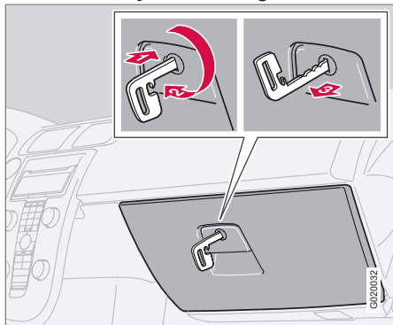
Beskyttelseslåsing aktiveres.
