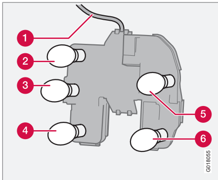
Pæreholder.
