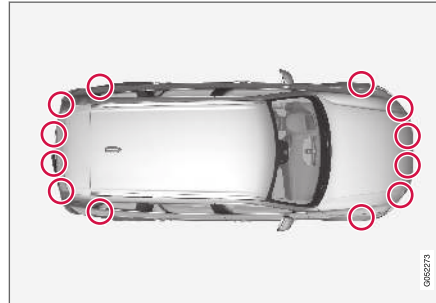
Positie van de sensoren 114 .
