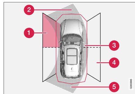
Gebieden waarbinnen de parkeersensoren obstakels kunnen ontdekken 121 .
