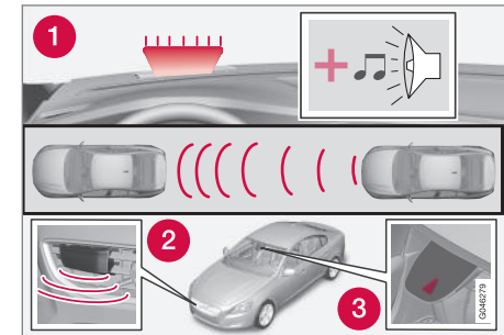
1. Témoin d'avertissement et répéteur acoustique de l'anticipation de collision 6 .
