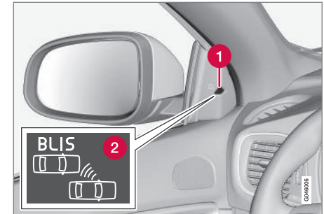
Positie BLIS-lampje 24 .
