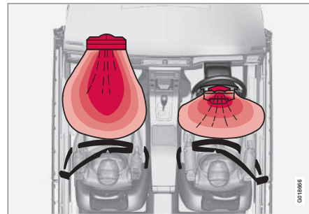
Κάτοψη συστήματος αερόσακων, δεξιότιμο αυτοκίνητο.
