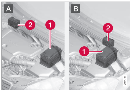
A : voiture à conduite à gauche. B : voiture à conduite à droite. (1) Batterie de démarrage 16 (2) Batterie d'appoint.
