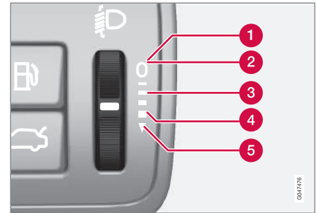
Duimwielstanden bij uiteenlopende belading.
