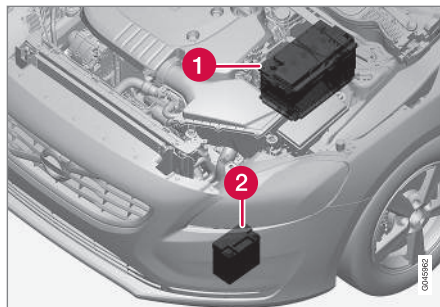
(1) Startaccu 17 (2) Hulpaccu
