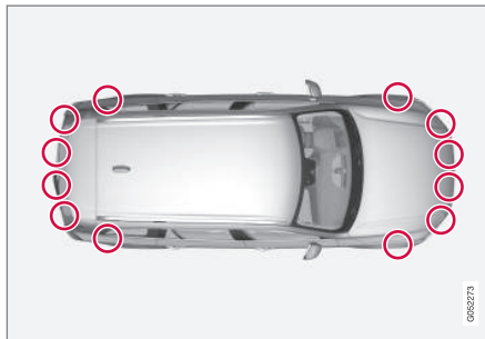
Posizione dei sensori PAP 29 .
