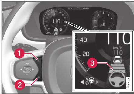
Aikaetäisyyden säädin 67 .
