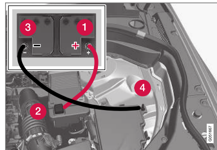
Aansluitpunten voor de startkabels.
