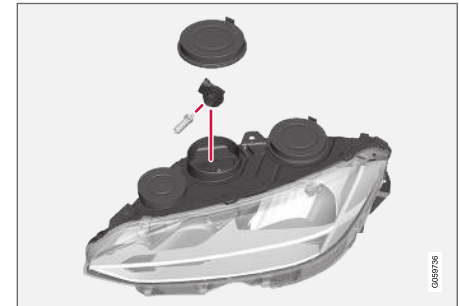
Linker koplamp.
