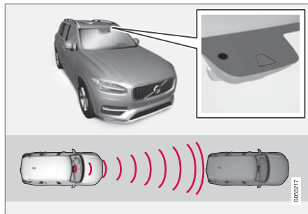
レーダーユニットの位置 80
