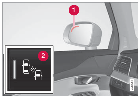
BLIS ランプの位置 85
