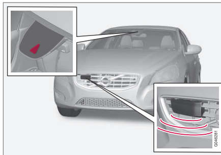
Αισθητήρας κάμερας και αισθητήρας ραντάρ 22 .
