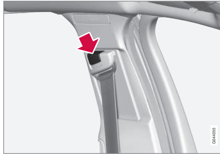
Ajuste vertical do cinto de segurança. Pressione o botão e desloque o cinto na vertical. Coloque o cinto o mais alto possível, sem que o mesmo entre em contacto com o pescoço.
