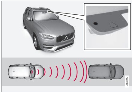
Umieszczenie modułu radarowego 14 .
