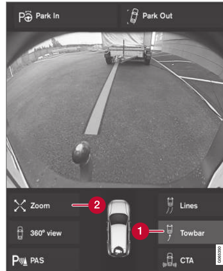
Anhängerkuppelung mit Hilfslinie 115 .
