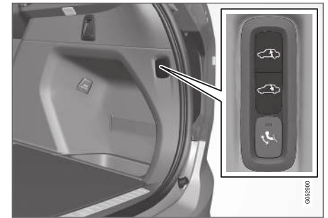
Comando per abbassamento/sollevamento del retrotreno.
