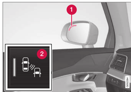
Posizione della spia BLIS 84 .
