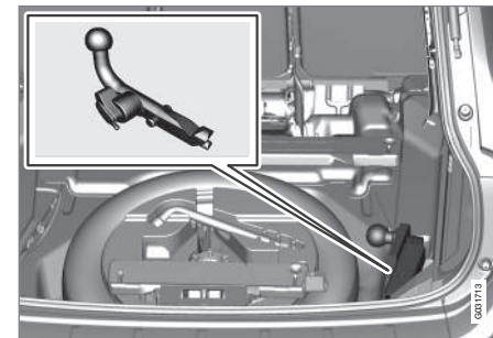
Compartimentos para arrumação do engate de reboque.
