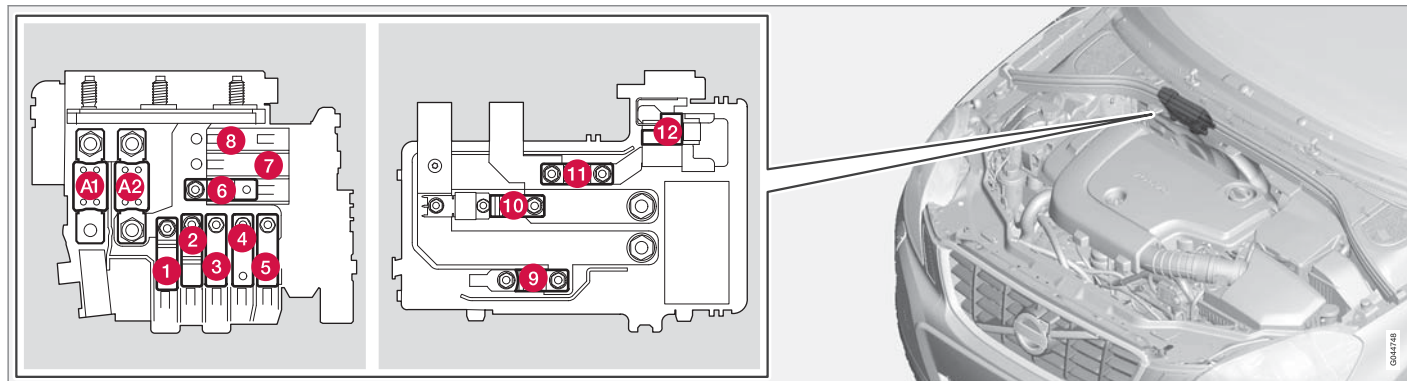
エンジンルームのコールドゾーン内のヒューズの位置
