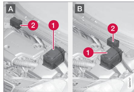
A：左ハンドル車。B：右ハンドル車。1. メインバッテリー 16 2. 補助バッテリー。
