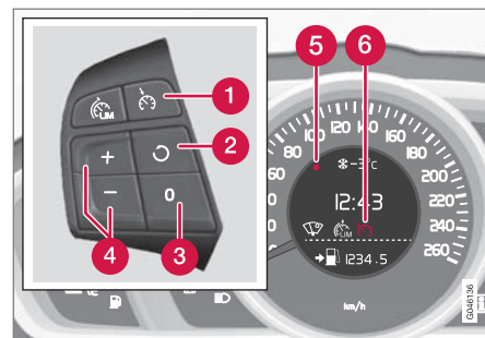
速度リミッター 装 備 6 の車両のステアリングリモコンとインフォメーション・ディスプレイ
