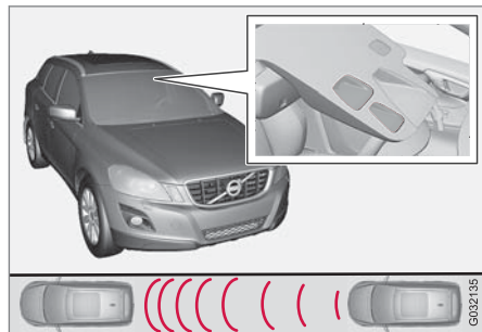
レーザーセンサーの送信/受信ウィンドウ 16
