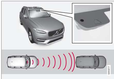
레이더 유닛의 위치.
