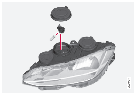
좌측 전조등.
