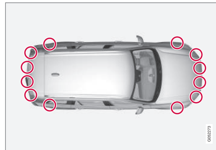
Pysäköintitunnistimien sijainti 24 .
