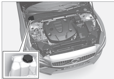
냉각수 탱크.
