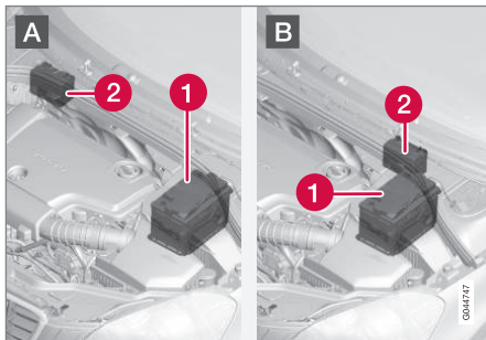
A: Samochód z kierownicą po lewej stronie. B: Samochód z kierownicą po prawej stronie. (1) Akumulator rozruchowy 16 (2) Akumulator pomocniczy.
