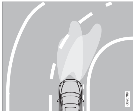
Fascio di luce fari attivi/non attivi.
