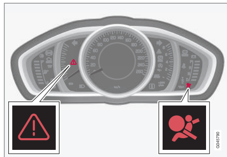
Triangolo di avvertimento e spia di allarme del sistema airbag (p. 34) nel quadro strumenti analogico.
