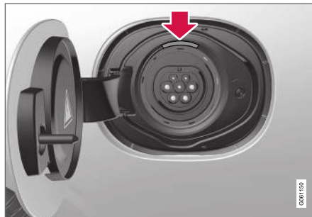
Localização da lâmpada de LED na tomada de entrada de carregamento do veículo.
