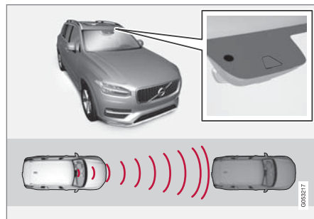
レーダーユニットの位置 82
