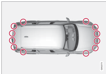
パーキングセンサーの位置 125
