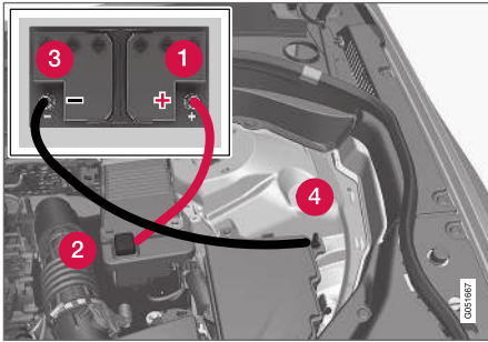
Käynnistyskaapelien kiinnityspisteet.
