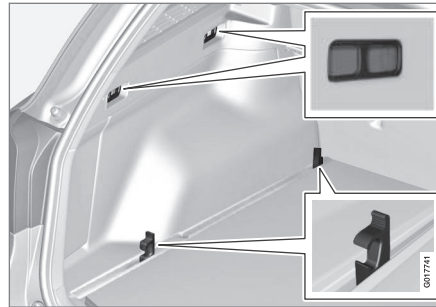
Fästpunkternas placering i lastutrymmet (med flyttbara lastsäkringskrokar).
