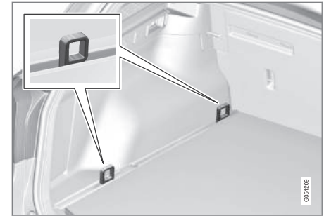
Fästpunkternas placering i lastutrymmet (med fasta lastsäkringsöglor).
