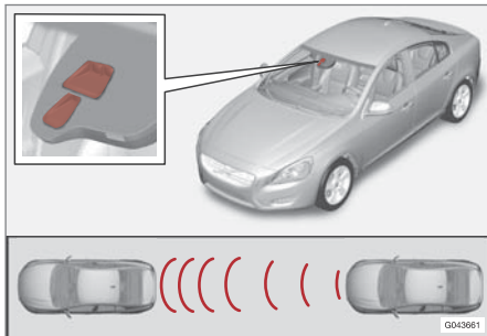
レーザーセンサーの送信/受信ウインド 14
